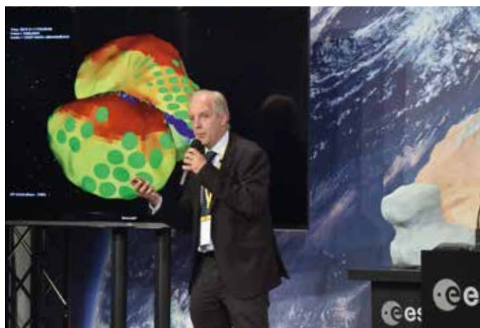
▲ Профессор Стефан Уладек на модели ядра кометы Чурюмова-Герасименко показывает возможные места посадки модуля Philae (зеленые кружки).
