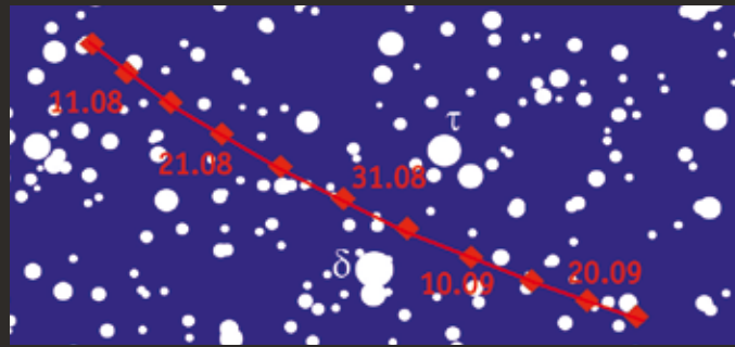
Видимый путь астероида Гармония (40 Harmonia) по созвездию Водолея в августе-сентябре 2014 г.
