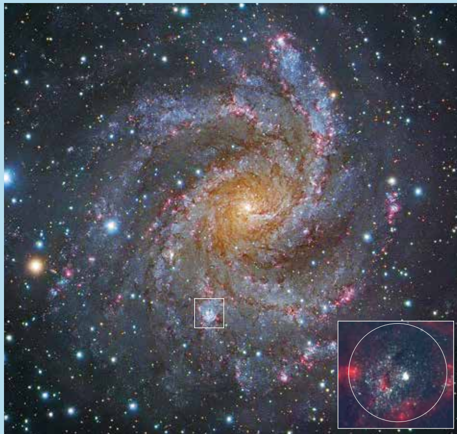
▲ Еще один пример возможной инженерной деятельности галактических масштабов — крайне странный молодой звездный комплекс в спиральной галактике NGC 6946. Снимок галактики получен телескопом «Субару» Японской национальной астрономической обсерватории, снимок фрагмента — звездного комплекса Ходжа — космическим телескопом Hubble. Помимо тысяч звезд высокой светимости, этот комплекс содержит гигантское молодое шаровое скопление (светлое пятно вблизи его середины) общей массой порядка миллиона солнечных и возрастом около 15 млн лет. Западный его край представляет собой правильную дугу протяженностью до 130°. Попытки объяснить происхождение этого комплекса естественными механизмами остаются безуспешными. Красный цвет соответствует областям ионизованного водорода, излучающего в линии H \alpha (656,3 нм).
