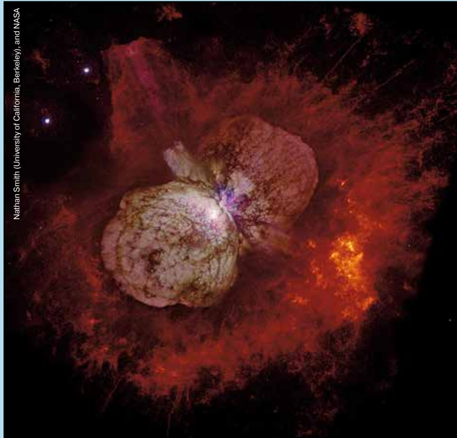
▲ Этот впечатляющий «портрет» системы η Киля составлен из снимков, сделанных Широкоугольной и планетарной камерой WFPC2 орбитального телескопа Hubble в сентябре 1995 г. в красной области видимого спектра и ближнем ультрафиолетовом диапазоне. 160 лет назад эта система пережила грандиозную вспышку, во время которой она стала вторым по яркости звездообразным объектом неба (после Сириуса). Вспышка была следствием мощного взрыва, сопровождавшегося выбросом в противоположные стороны двух огромных газовых облаков и тонкого диска в плоскости, перпендикулярной их оси. Все эти гигантские массы пыли и газа разлетаются со скоростью около миллиона километров в час.
