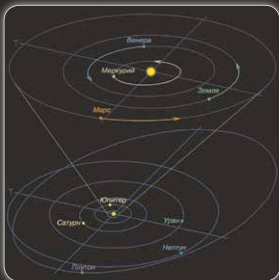
Положения планет на орбитах в сентябре-октябре 2014 г.
